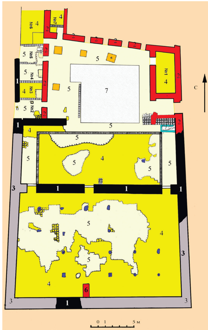
2-расм. Шаҳар марказидаги қазимиша (Қазимиша №6, 2005, 2007, 2009 йй). XVIII-XX асрлар бошига оид Жомъе масжиди тарҳи. 1. Пишган ғишдан қурилган пойдевор қолдиқлари. 2. Пахса девор қолдиқлари. 3. Бузилган девор излари. 4. Пишган ғишдан терилган пол. 5. Полнинг бузилган қисми. 6. Меҳроб. 7. Қазилмаган ҳудуд.
